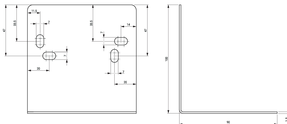
Rysunki wymiarowe
