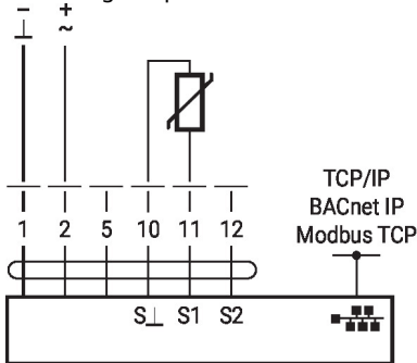
Aansluiting van passieve sensoren
