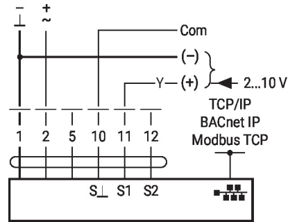
Schakelcontactverbinding
