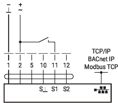
Schakelcontactverbinding
