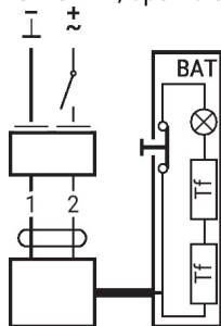
AC/DC 24 V, open/dicht
