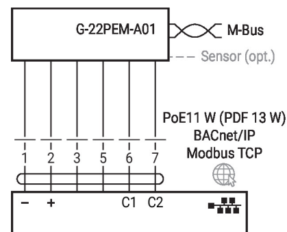
M-Bus in parallelo a Modbus TCP o BACnet/IP con PoE
