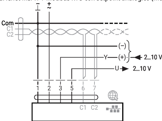
MP-Bus, alimentazione tramite alimentazione a 3 fili
