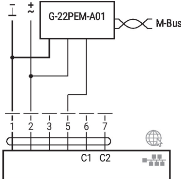
M-Bus con convertitore
