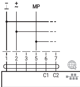
M-Bus con convertitore
