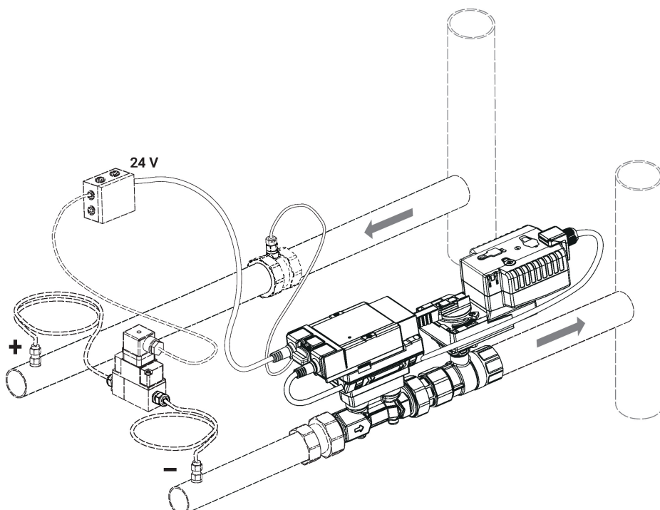
Energy Valve con accessori Sensore di pressione differenziale 22WDP-11.. Raccordo EXT-EF-..F Pezzo a T con pozzetto A-22PE-A0..
