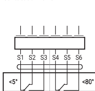
Contact auxiliaire
