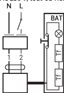
AC 230 V, tout-ou-rien
