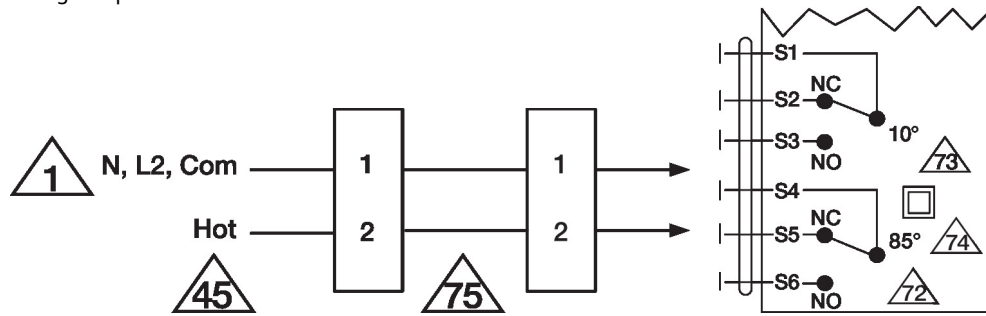
Câblage en parallèle des servomoteurs
