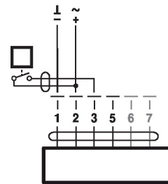
Connexion avec contact de commutation
