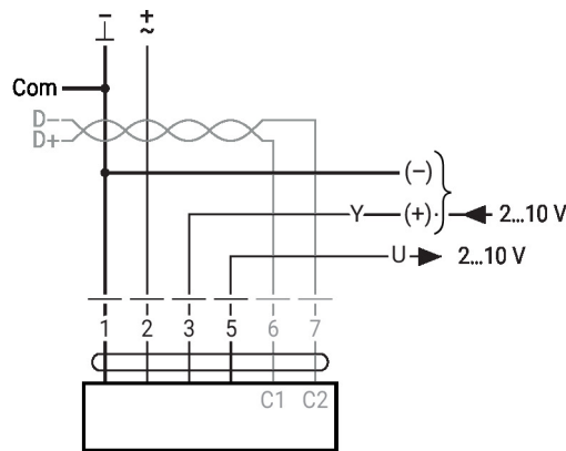
Modbus RTU / BACnet MS/TP con valor de referencia analógico (funcionamiento híbrido)
