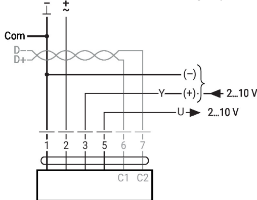
MP-Bus
