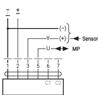
MP-Bus
