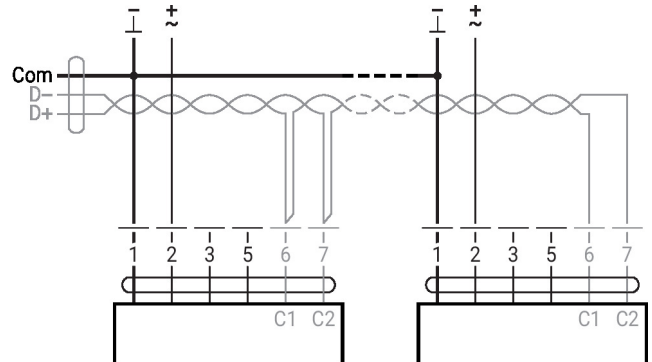
BACnet MS/TP / Modbus RTU
