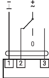
AC/DC 24 V, 3-Punkt
