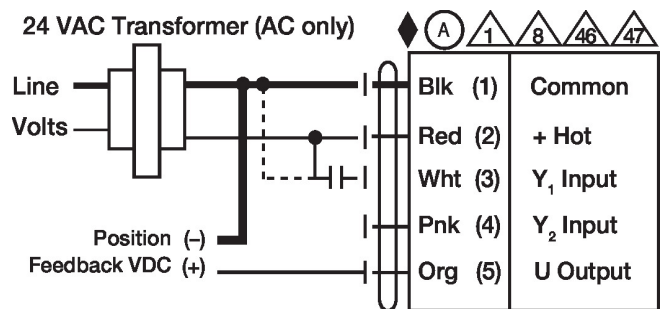
Commande PWM
