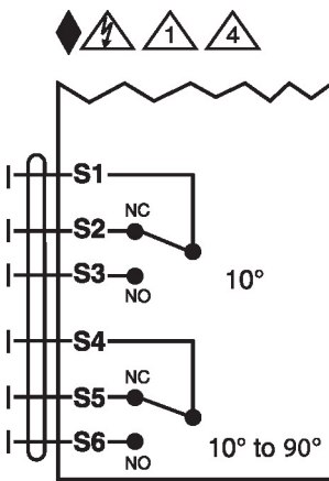
Interrupteurs auxiliaires
