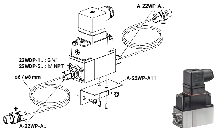
Differenzdrucksensor Wasser – 22WDP-11.. von Belimo
