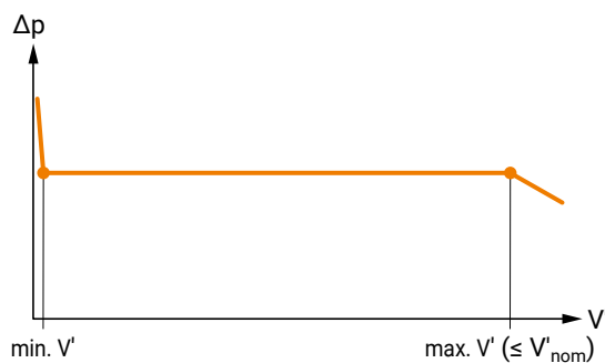
Arbeitsbereich Differenzdruckregelung
