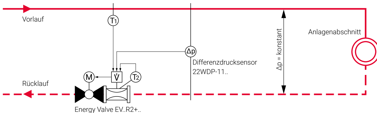
Differenzdruckregelung mit Energy Valve
